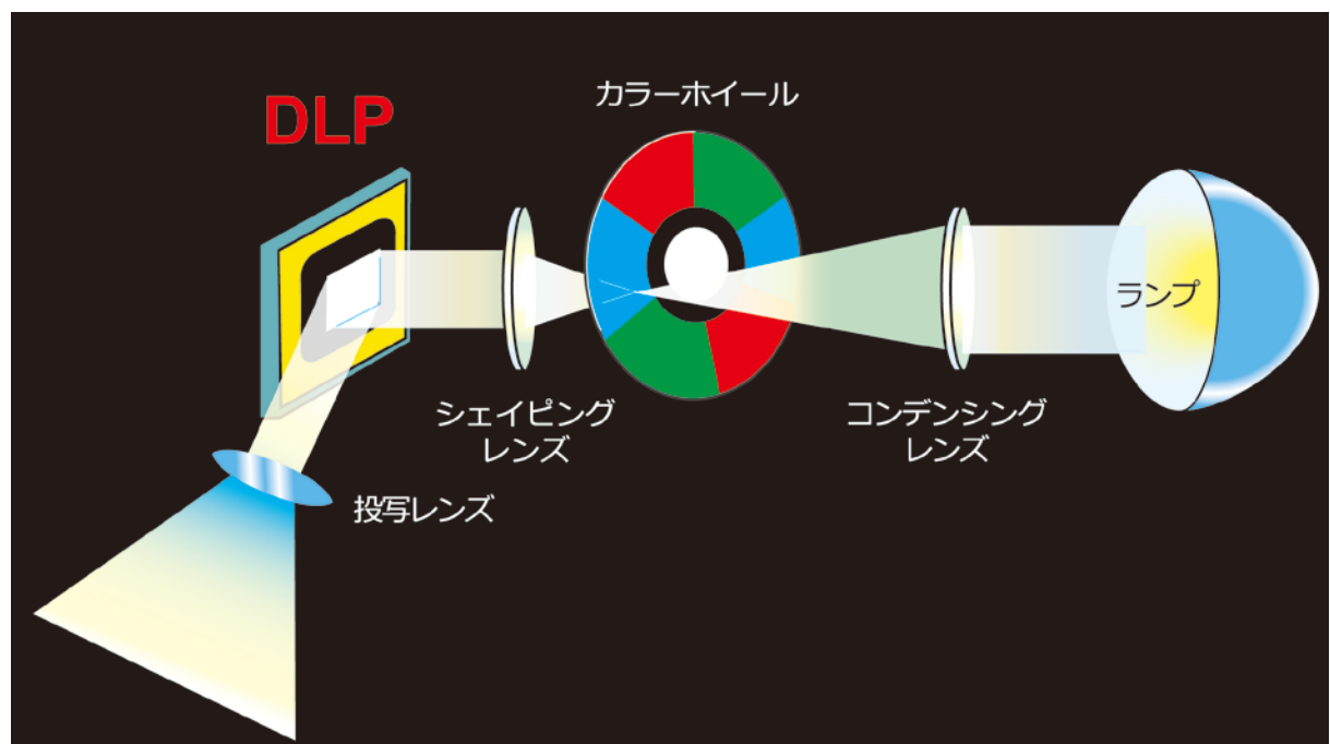
DLP の仕組み
