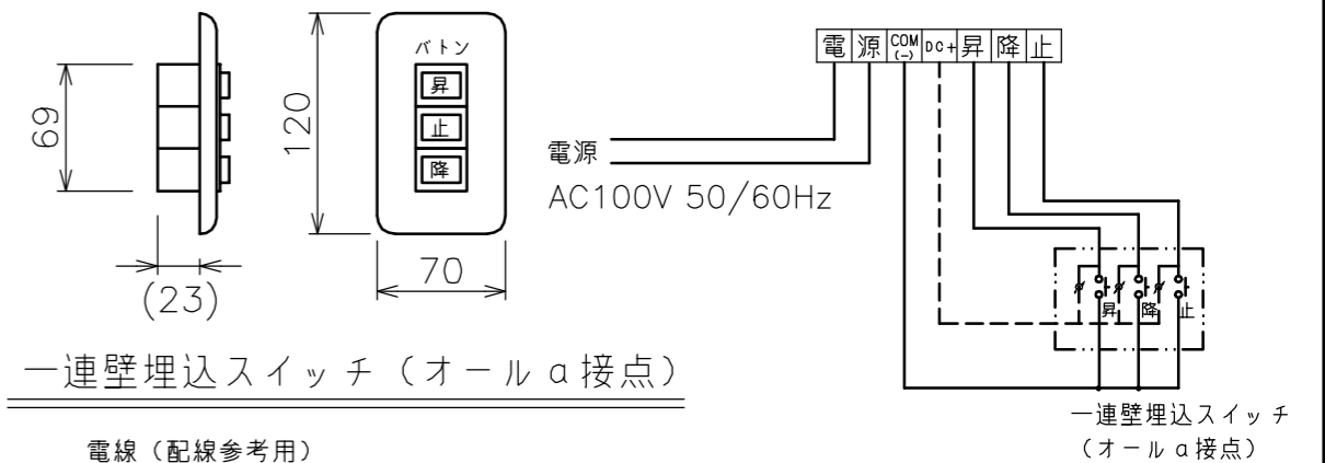
結線図
