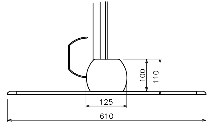
a部拡大図 (S=1/5)
