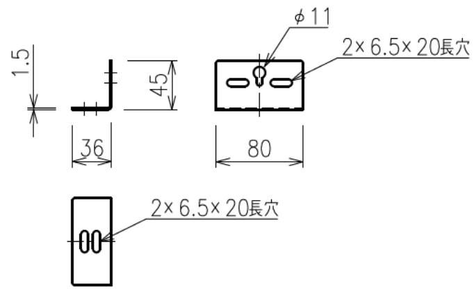
スクリーン取付金具詳細 S=1:5
