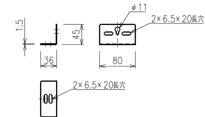
スクリーン取付金具詳細 S=1:5
