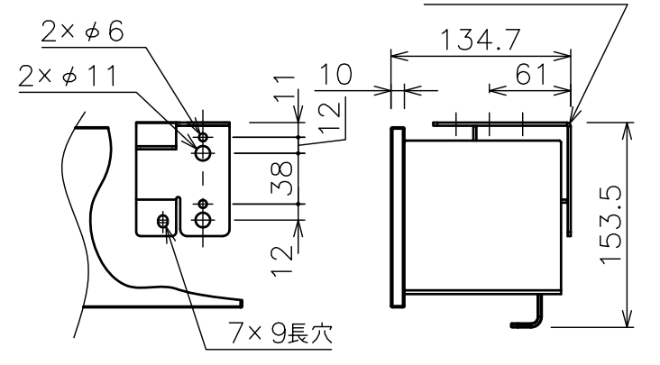
サイドブラケット詳細図(S=1/5)
