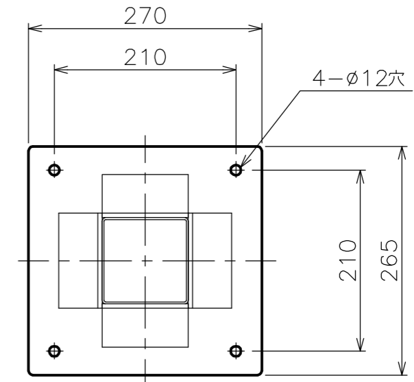
矢視 A - A <ハンドル側>
