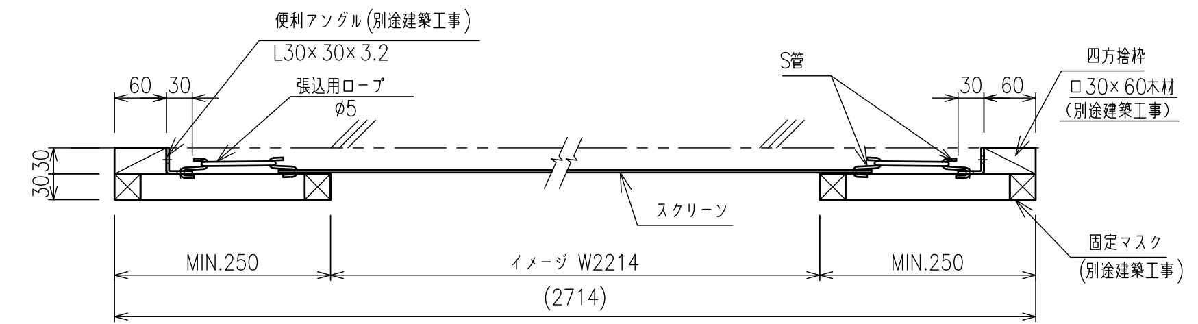
矢視 A - A
