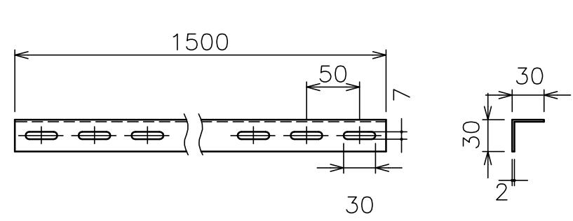
スクリーン取付金具詳細 (s=1/5)
