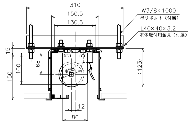
矢視 A - A
