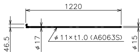
フック棒HK-1200A 質量0.11kg
