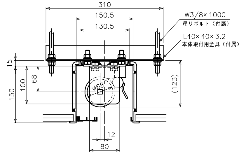
矢視 A - A
