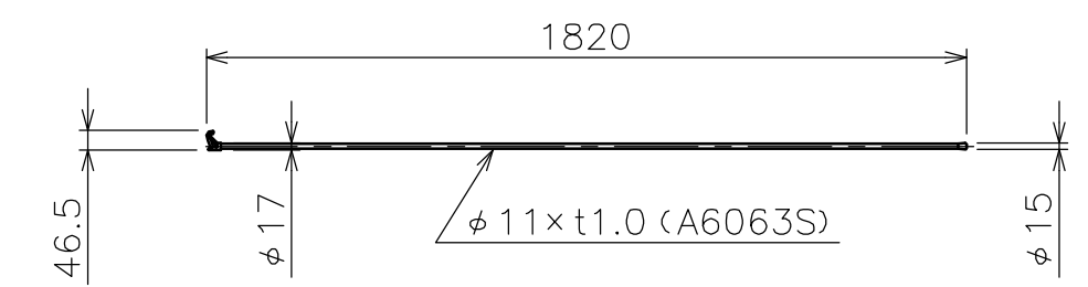
フック棒HK-1800A 質量0.16kg
