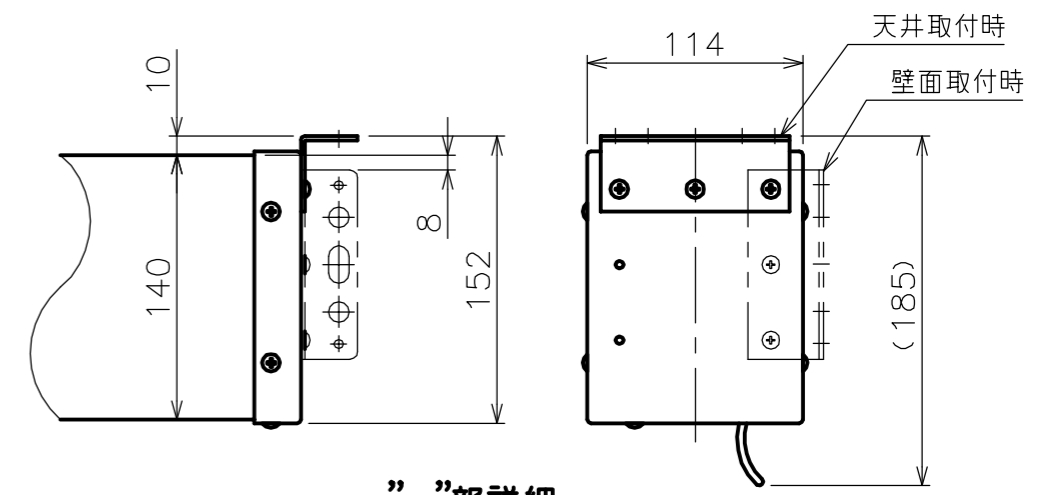
”a”部詳細
