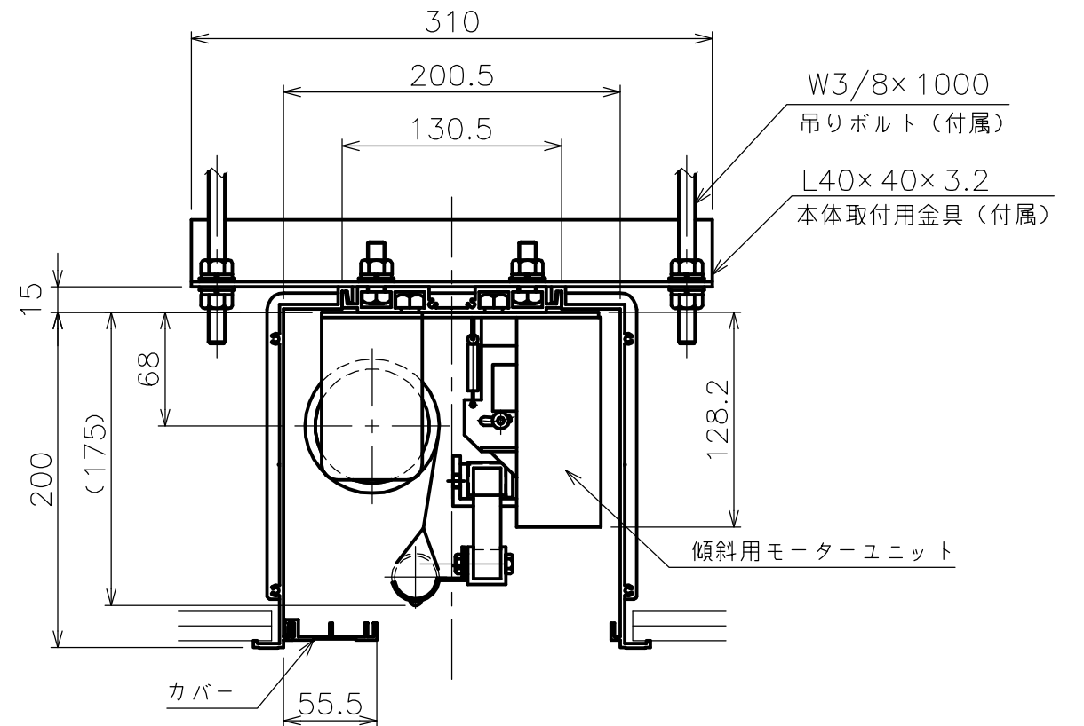
矢視 A - A
