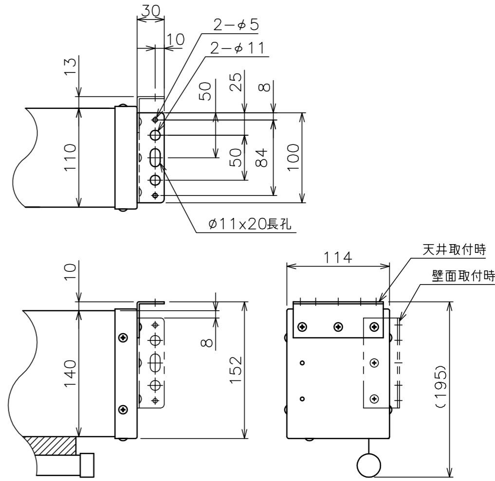
”a”部詳細
