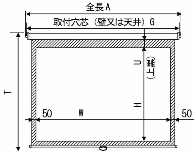
■前から見た図
