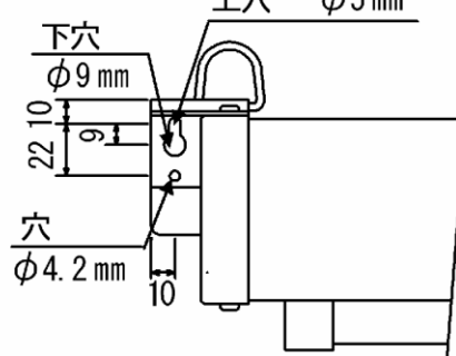
■前から見た図
