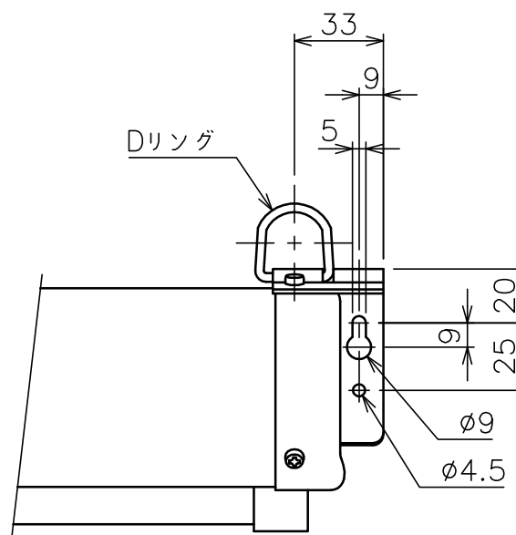
”a” 部詳細
