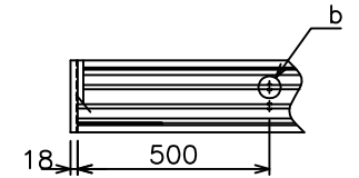
矢視 B
