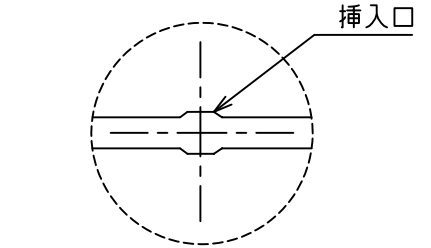
b部 M10ボルト挿入口拡大図
