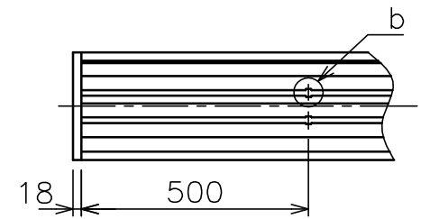
矢視 B
