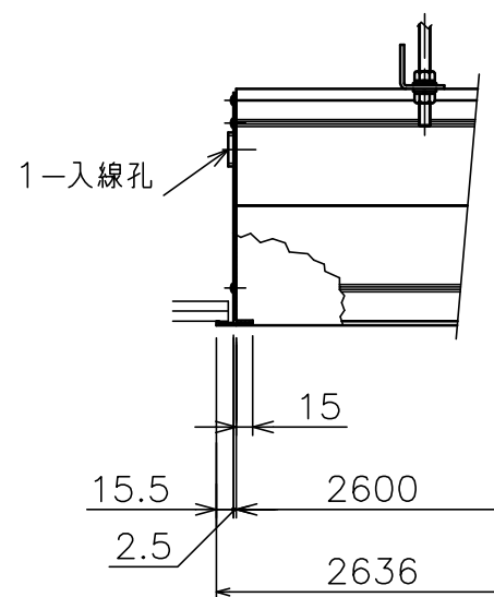
”a”部詳細
