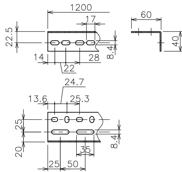
スクリーン取付金具詳細
