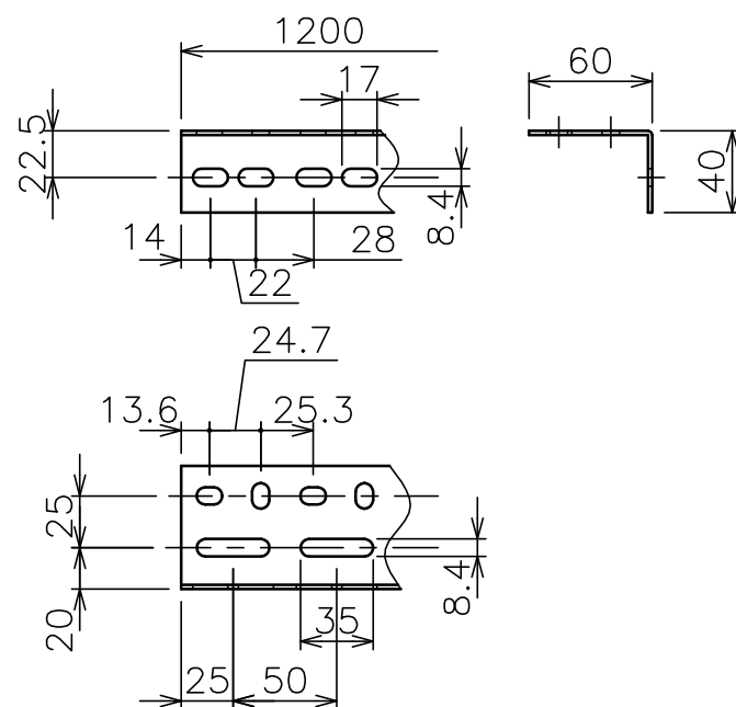
スクリーン取付金具詳細
