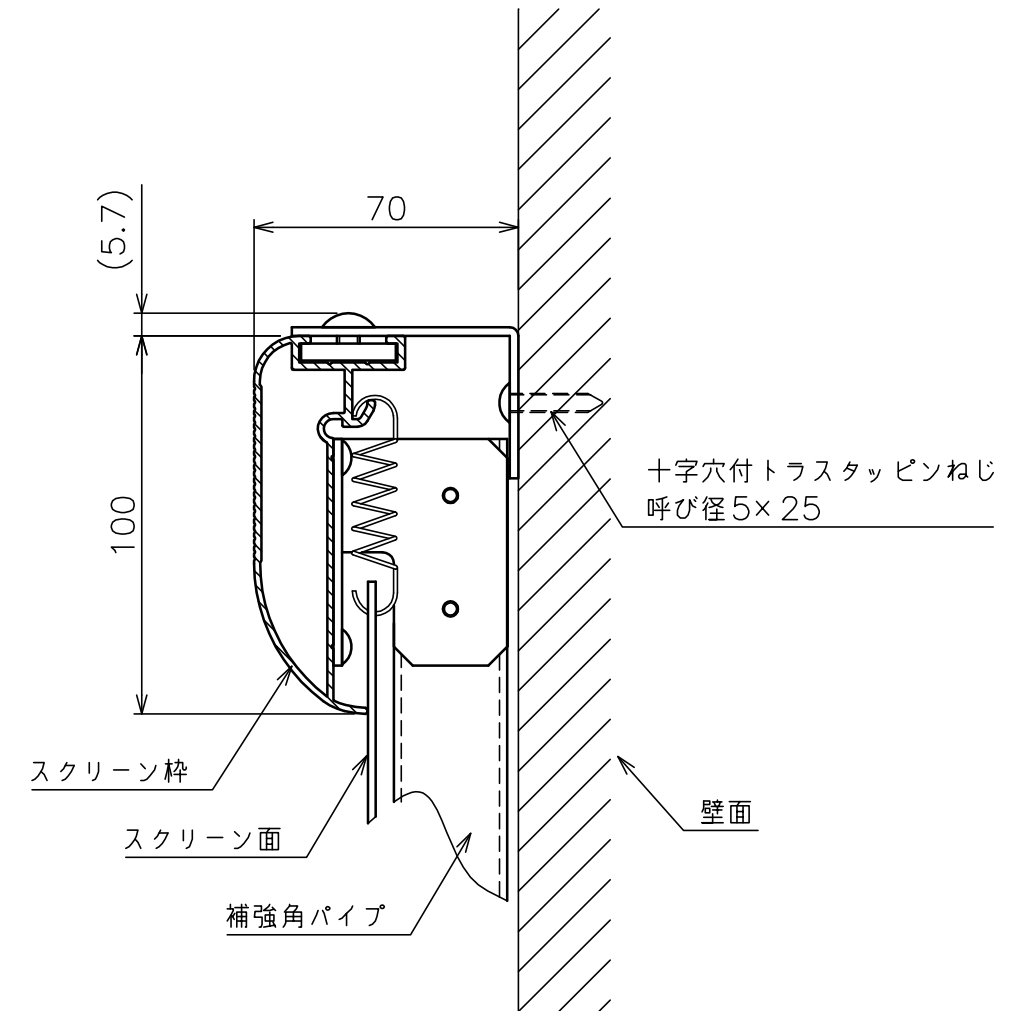
断面A-A
