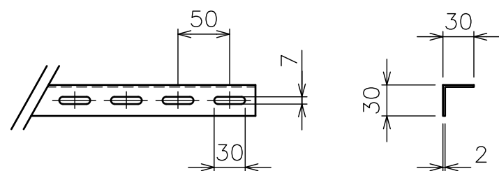
スクリーン取付金具詳細
