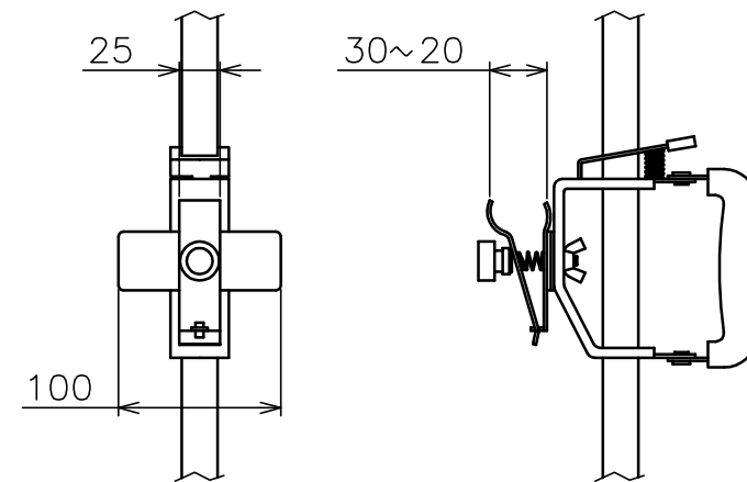
クリップ部詳細 (SMHタイプ用)
