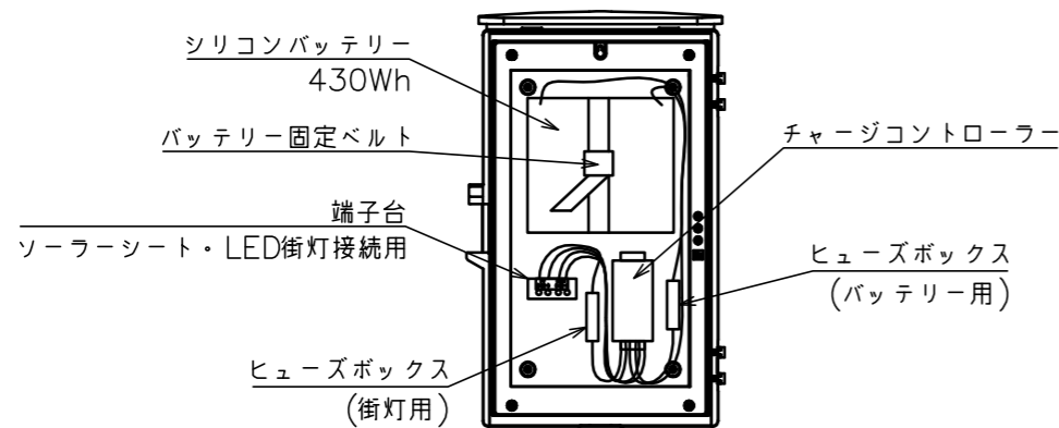
バッテリー収納ボックス (内部レイアウト)
