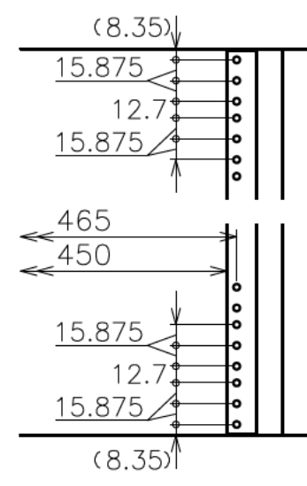
EIA 詳細図
