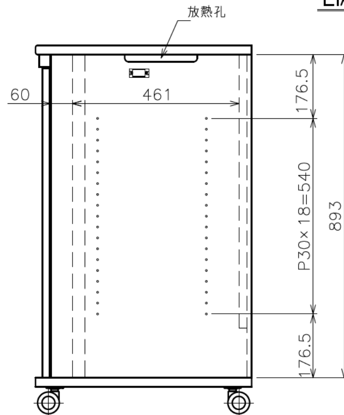
EIA 詳細図
