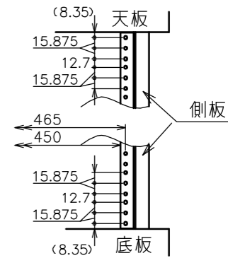
EIA金具 詳細図
