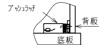
a部詳細
