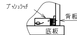
a部詳細
