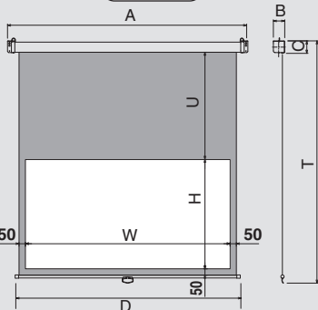
外形寸法図 (手動/SMC)
