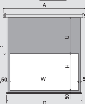
外形寸法図 (電動/SEC)
