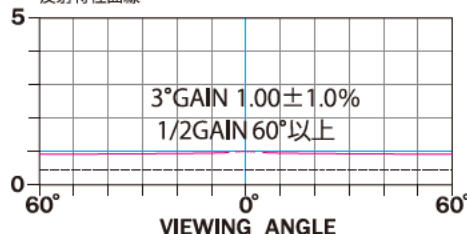
反射特性曲線
